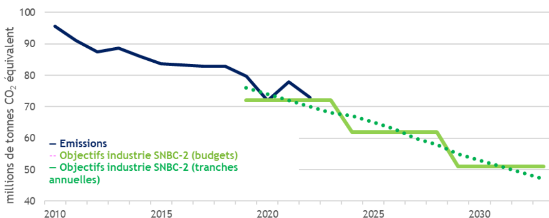
Evolution des émissions dans l'air de CO 2 e du secteur de l'industrie manufacturière et construction en France (Métropole et Outre-mer UE)
