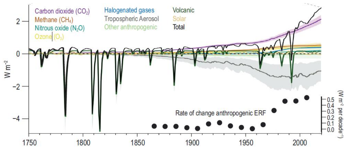
Figure : L'augmentation du forçage radiatif effectif depuis la fin du XIXe siècle est principalement due au réchauffement des GES et au refroidissement des aérosols. (Giec, 2021, Technical summary, Vol. 1) Le CO 2 est lié principalement aux combustions industrielles et domestiques ainsi qu'aux transports. Le CH 4 est en majorité lié aux pratiques agricoles : par exemple l'élevage et la riziculture. Le N 2 O a une origine principalement agricole avec l'usage des fertilisants minéraux et d'origine organique (engrais, fumier, lisier).
