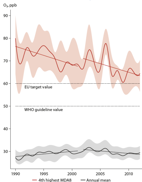
Evolution des pics de concentration d'ozone (4ème plus haut niveau quotidien des concentrations en ozone moyennes sur 8 heures) et les concentrations moyennes annuelles sur les 54 stations de surveillance EMEP avec une couverture de données satisfaisante.
