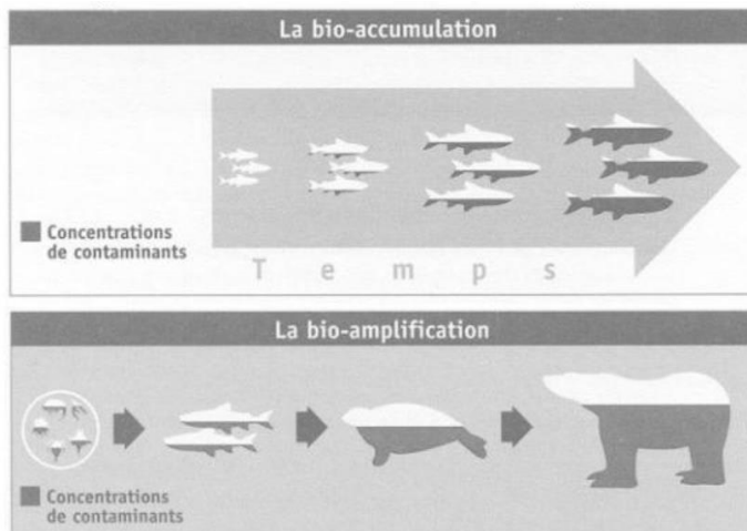
Figure : La bio-accumulation et la bio-amplification (Observatoire midi Pyrénées)
