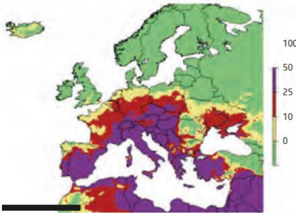
Nombre de jours où la moyenne journalière sur 8 heures a dépassé le seuil de 100 µg/m 3 (valeur guide de l'OMS) en 2017 (source : Copernicus Atmosphère Services).
