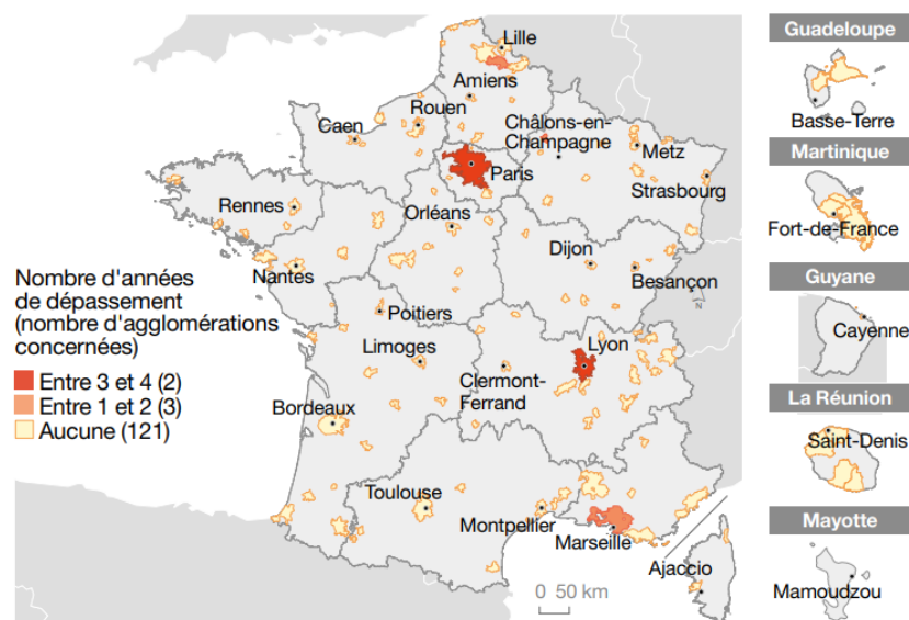
PM_{2,5} (période 2009-2021)
