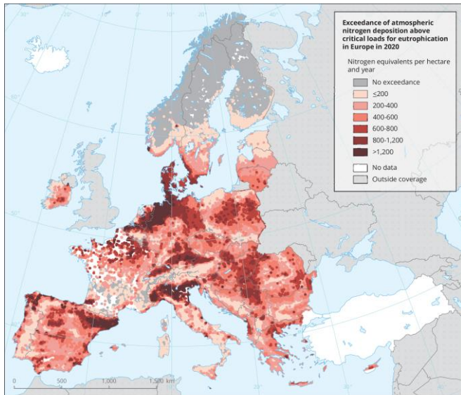
Figure : Dépassement des dépôts atmosphériques d'azote au-dessus des charges critiques pour l'eutrophisation en Europe en 2020
