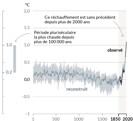
Changement de la température à la surface du globe (moyenne décennale) reconstruite (1-2000) et observée (1850-2020), (GIEC, 2021, Résumé pour les décideurs, AR6)
