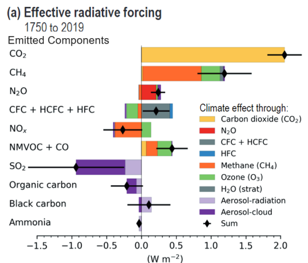
Figure : Forçage radiatif des composés (IPCC- AR6-2021).
