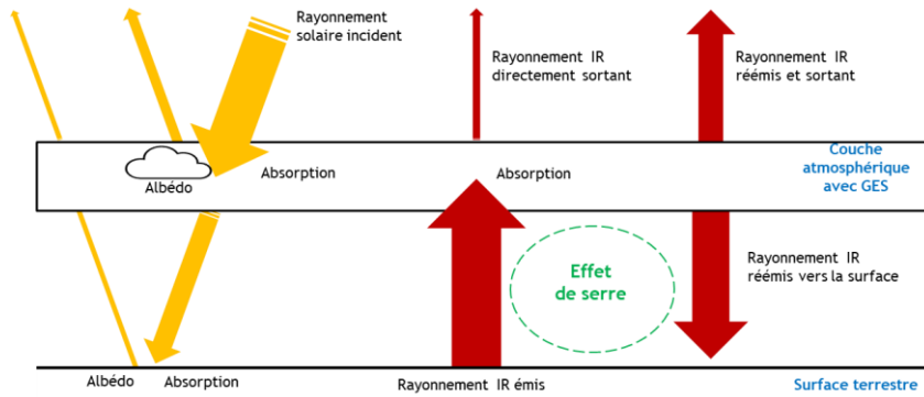
Figure : Bilan radiatif terrestre (Citepa)
