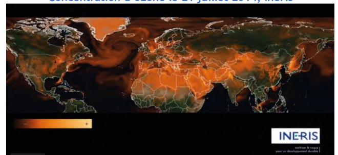
Concentration d'ozone le 21 juillet 2014, Ineris
