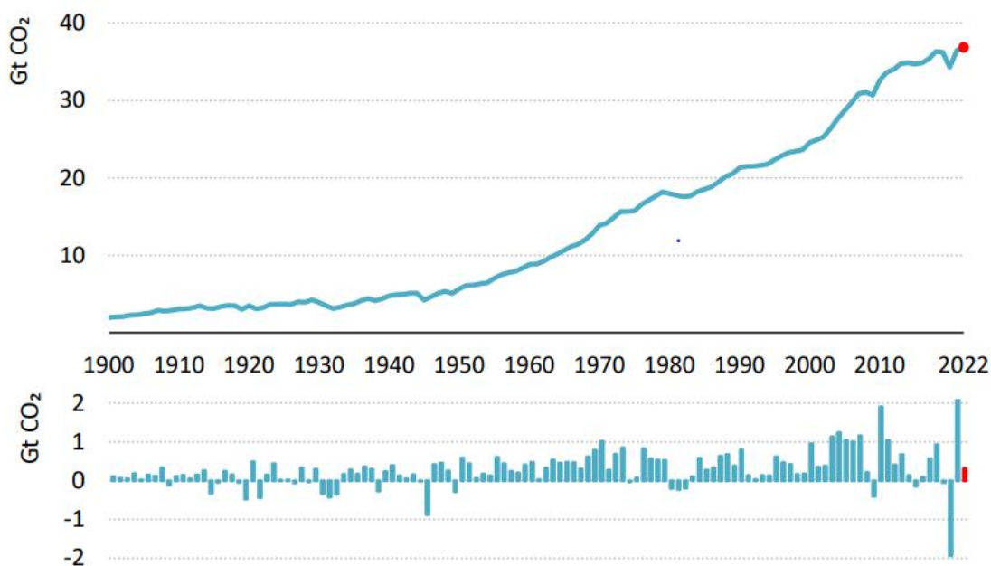
Emissions mondiales de CO 2 liées à l'énergie et leur évolution interannuelle 1900-2022 (en Gt CO 2 )
